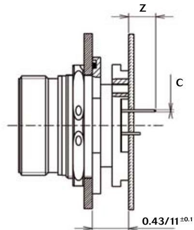
Jam nut double flange receptacle 8D8711
